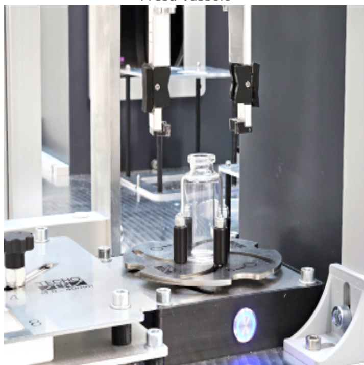
Presa da autocentrante
